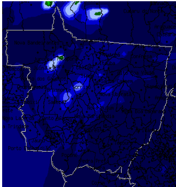
Fonte: CATT- BRAMS - CPTEC/INPE Data: 05/09/2013. Material Particulado. Horário da imagem 12:00 h.
