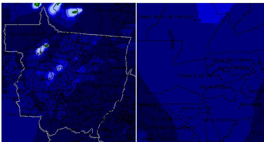
Fonte: CATT- BRAMS - CPTEC/INPE Data: 26/09/2013. Material Particulado. Horário da imagem 12:00 h.
