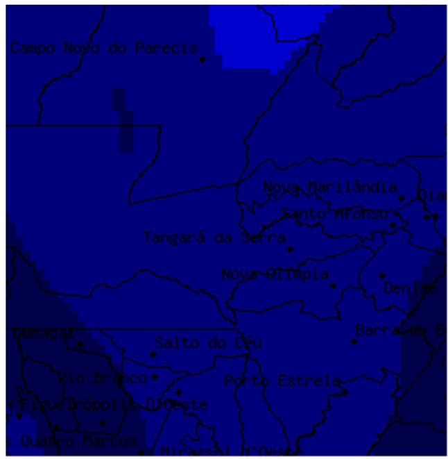
Fonte: CATT- BRAMS - CPTEC/INPE Data: 18/02/2014. Material Particulado. Horário da imagem 12:00 h.
